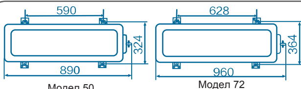
Монтажни размери на външното тяло (мм)
