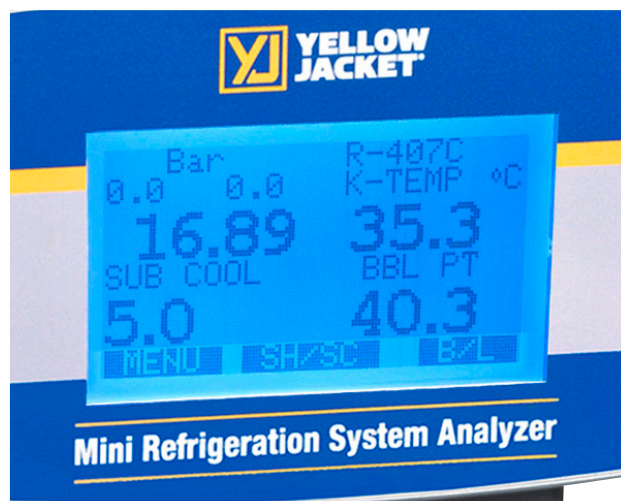
bar - Subcool
